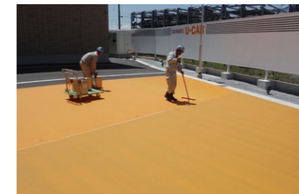
2. 吹付2層目
