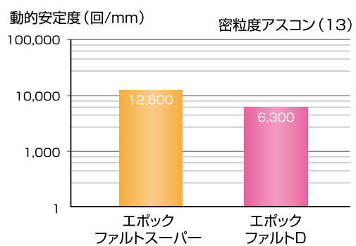
図 ホイールトラッキング試験による動的安定度の比較
