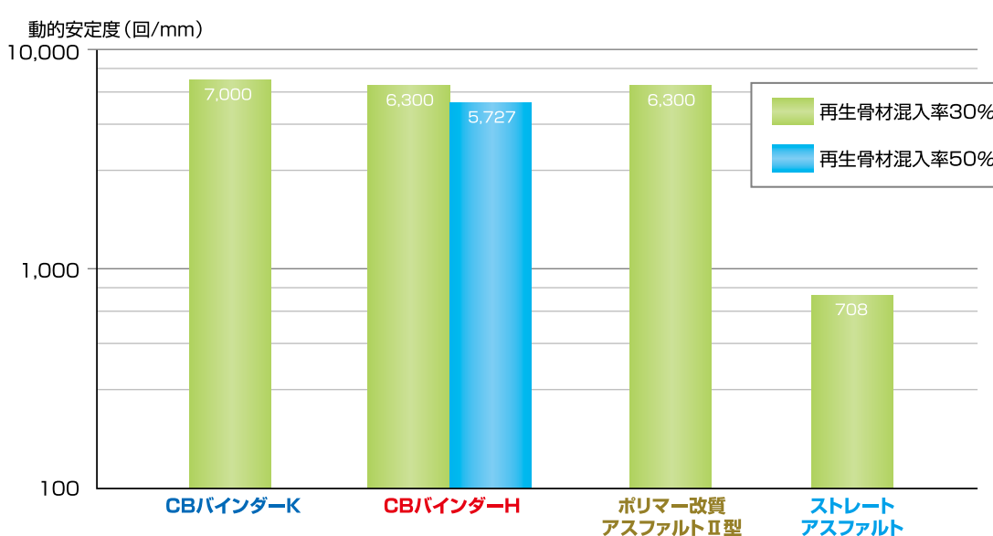
図 再生ポリマー改質アスファルトを使った再生加熱アスファルト混合物の動的安定度の比較例
